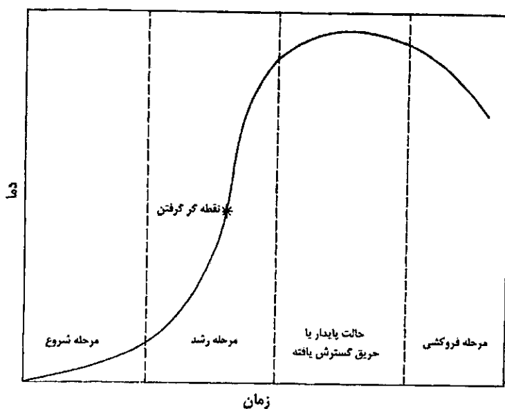
شکل پ ۲-۳: منحنی استاندارد رشد آتش‌سوزی
